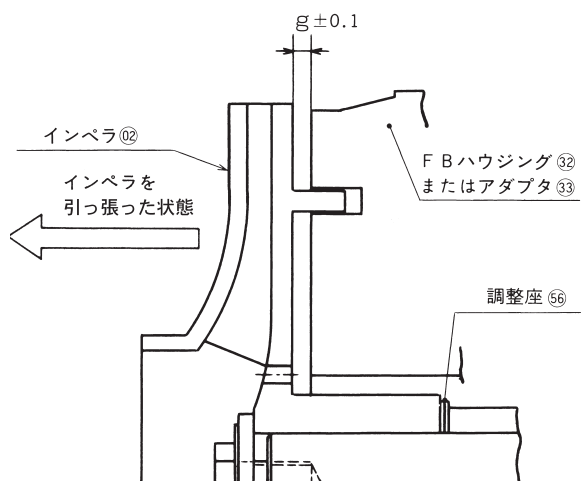
図11 (標準品)
